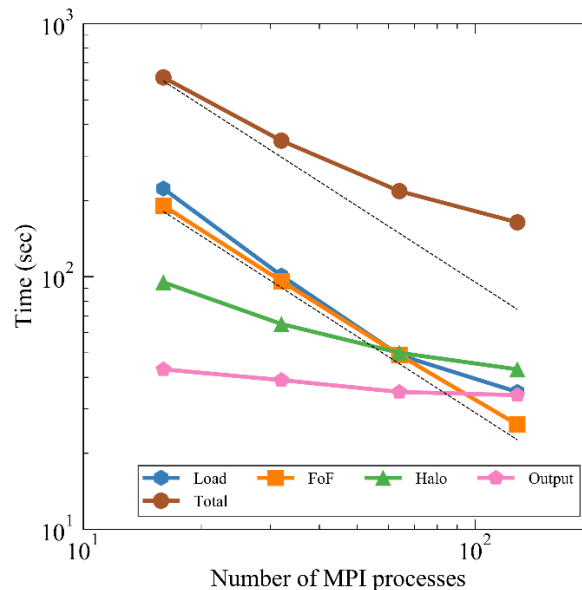
図 3-1-1: ハロー検出ソフトウェアの並列性能。富岳上で 1024^3 粒子を用いたテスト計算の結果である。Load は粒子データの読み込み、FoF はハローグループの検出、Halo はグループから個別のハロー検出、Output はデータの出力を表す。
