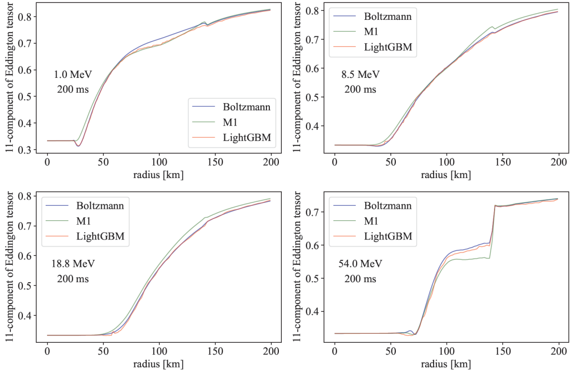
図 5-2-1 : バウンス後 300 ms のデータを再現するように訓練した AI モデルで、バウンス後 200 ms のデータを出力した結果。エディントンテンソルのフラックス方向成分の動径分布を書いており、青、緑、赤の線はそれぞれ正答、慣習的な関係式の結果、今回の AI モデルの結果に対応する。4 枚の図はそれぞれ違ったニュートリノエネルギーでの動径分布を表す。緑の慣習的モデルより赤の AI モデルのほうが青の正答をよく再現できている。
