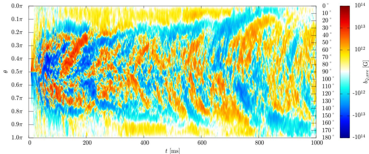
図 5-3-1: ブラックホールを中心とした半径 100km の球上で評価した、平均トロイダル磁場のバタフライダイアグラム。ディスク内部 (90 度の赤道面付近) で周期的に逆極性の磁場が生成されていること、生成された磁場が極 (0 度、180 度) 方向に浮上していることが確認される。また、浮上した磁場が極付近の磁場極性を反転させていることも確認される。
