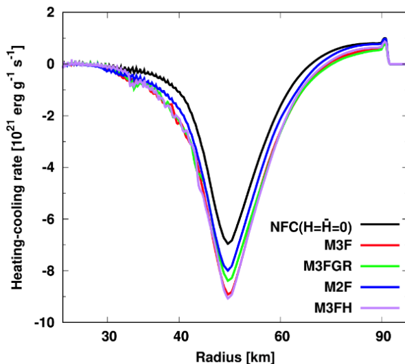
図 5-2-3 : ニュートリノ冷却及び加熱率の動径分布。黒線（その他の色線）が古典的（量子運動論的）ニュートリノ輸送シミュレーションの結果。本結果は、ニュートリノフレーバー変換が爆発メカニズムに影響を与える事を示している。
