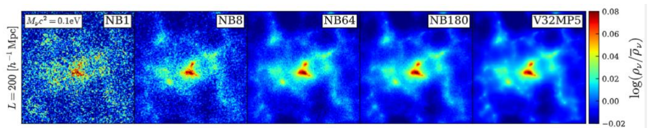
図 3-2-1: ニュートリノを Vlasov シミュレーションで計算した結果(一番右のパネル)と N 体シミュレーションを用いて計算した結果(粒子数の少ない順に NB1、NB8、NB64、NB180)の比較。粒子数が少ない場合はショットノイズの影響が大きいことが分かる。
