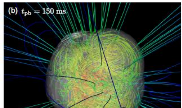
図 5-2-2 : 超新星爆発の爆発波面のスナップショット。磁場の形状を磁力線でその強さを色で表している。弱自転があることにより、極めて強い磁場ができている。
