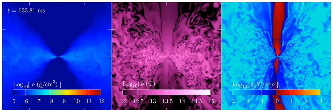
図 5-3-2: 400km スケールの xz 平面スナップショット。ブラックホールは中心に位置しており、その回転軸は z 方向 (縦軸方向)。左からそれぞれ静止質量密度、磁場強度、磁化パラメータ。磁化パラメータを見ると磁場優勢な領域の形成が確認される。
