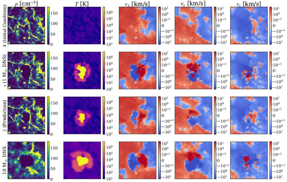
図 3-3-1: 超新星爆発後の周囲のガスの時間進化について、シミュレーション結果と機械学習による予測の比較。上段から、初期条件、高分解能のシミュレーションの結果、機械学習による予測、低分解能のシミュレーションの結果。左から、ガスの密度分布、温度分布、速度分布 ( x , y , z 方向)。
