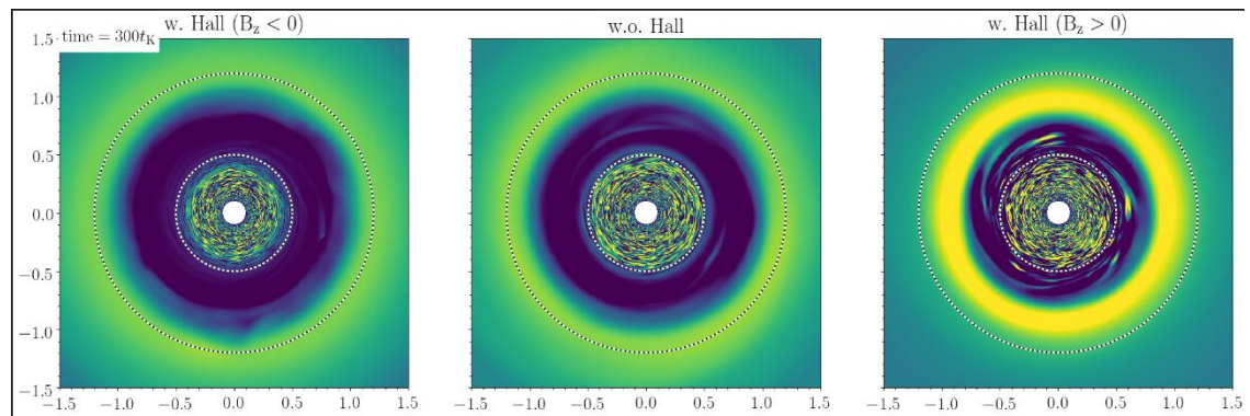
図 4-2-1：円盤赤道面の縦磁場分布。ホール効果を考慮しないシミュレーション(中図, Iwasaki et al. in press)とホール効果を考慮したシミュレーション(左図：円盤角運動量と初期縦磁場が反平行な場合, 右図：円盤角運動量と初期縦磁場が平行な場合)を示す。
