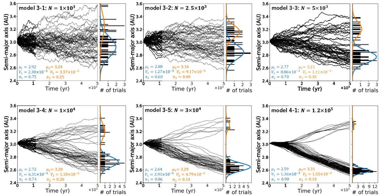
図 4-3-1: PDM による原始惑星の軌道長半径の進化。左上から右下にむけて、面密度は一定で微惑星の粒子を増やしている。それぞれのパラメータで複数のランを行い、5000 年後の軌道長半径の分布と、ガウシアン 2 つによるフィットも示す。
