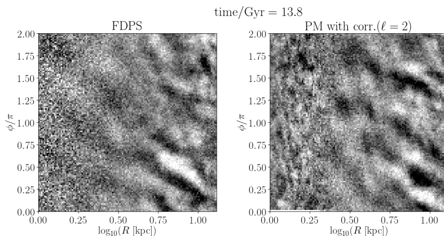
図 4-1-1: 10^7 体の恒星粒子を使った銀河円盤シミュレーションのテスト計算の結果。色は星面密度の方位角平均からの差を表す。左図がツリー法を用いた (FDPS, Iwasawa et al. 2016) で、右図が PM 法 (Athena++) を用いた結果。右斜め下に傾いた筋状の構造が渦状腕に対応する。 \log_{10}(R[\text{kpc}]) < 0.25 の構造で見られるツリー法と Particle-Mesh 法の結果の違いは、PM 法の分解能の影響と考えている。
