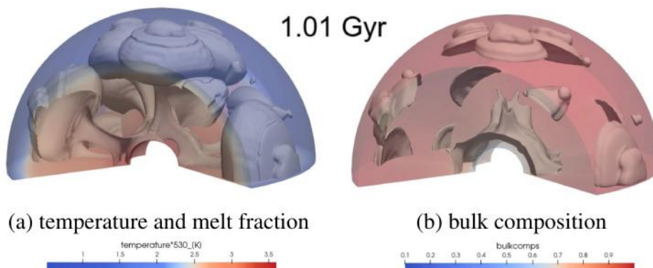
図 6-2-3: 火成活動を伴うマントル対流の 3 次元シミュレーションにより、月内部のマグマ上昇とそれに伴う玄武岩（マグマ的物質）の移動を追跡した例。(a) 月内部の温度分布（色）と液相の体積分率が 1% となる位置（等値面）の分布。(b) 月内部の岩石組成（かんらん石成分の割合）の分布。赤色はかんらん岩質のマントルを表しており、等値面は玄武岩質のマグマの流入により、かんらん石成分が 90% を
