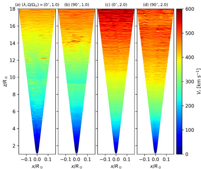
図 6-1-2: 太陽の 1 倍 (パネル a, b)、2 倍 (パネル c, d) の自転速度を持つ恒星風のシミュレーション結果。極域 (パネル a, c) と赤道域 (パネル b, d) でそれぞれ計算を実施した。カラーは恒星風速度のスライス [km/s]。
