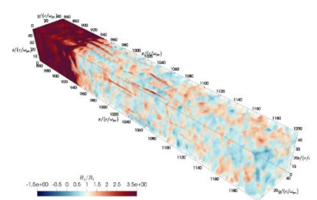
図 5-1-1: 相対論的衝撃波からの電磁波放射。色は磁場の変動成分の大きさを表す
