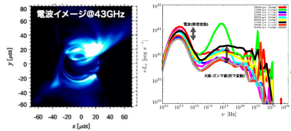
図 5-1-4 : (左) 電波イメージ、(右) 多波長スペクトル時間変動
