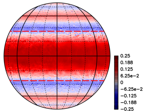
図 6-2-4：ガス惑星大気計算の 24000 回転時間経過後の惑星表面帯状風分布。赤が西風、青が東風、赤破線が内側境界の接円筒緯度を表している。風速は回転角速度と球殻の厚さで無次元化されている。
