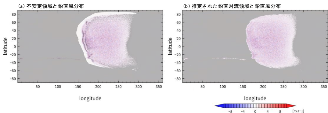
図 6-2-1: 火星大気高解像度計算による鉛直風分布 (色) と機械学習の結果。(a) の白抜き領域は温度場から計算した静的不安定な領域を表し、(b) の白抜き領域は学習モデルを使って推定した鉛直対流の領域を表す。
