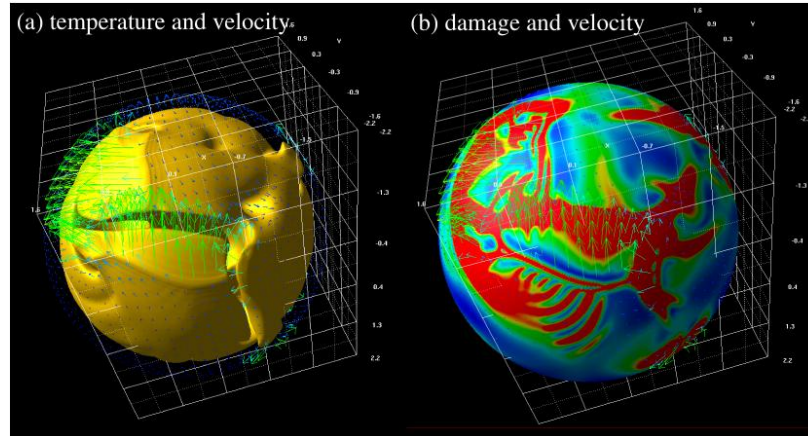
図 6-2-2: 応力履歴依存レオロジーをもつ高粘性流体の 3 次元球殻内熱対流シミュレーションの一例。(a) 球殻の最上部における流速（矢印）と高温の等値面の分布。(b) 流速（矢印）とダメージ（色）の分布。緑から赤色が過去に高い応力を受けて強く破壊された部分、青色は破壊されていない部分を示す。
