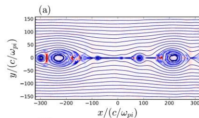
図 5-1-2: 電流密度と磁力線で表した磁気リコネクションの大規模発展
