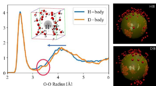
図5 核の量子効果を含む第一原理シミュレーションによって得られたプロトン周辺の構造。
