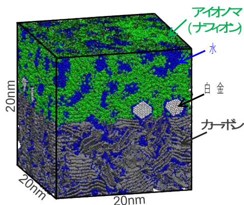
図3 100万原子系のモデル。白金を担持した炭素材料の上部に含水した高分子電解質膜が配置されており、電極界面を局所的にモデルしている。
