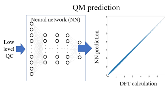
図6 機械学習(ニューラルネットワーク)モデルによるDFT計算の予測。通常のDFT計算と比較して10~1000倍程度高速に分子の電子状態プロパティを予測することが可能。
