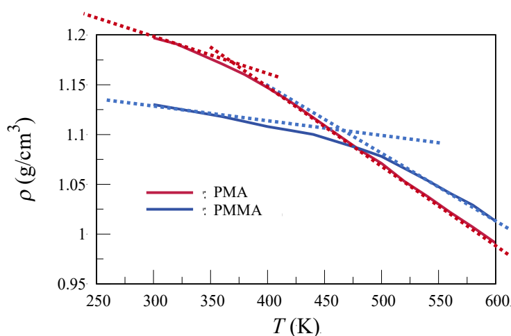
図 4. ポリメチルアクリレート (PMA) とポリメチルメタクリレート (PMMA) の各温度での密度。点線は高温領域と低温領域のフィッティング線。ガラス転移温度 ( T_g ) はフィッティング線の交わった点に対応する。
