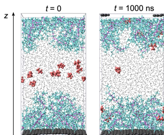
図1. ポリマーブラシへの吸着のMDシミュレーション。基板であるグラフェンの炭素原子を黒、吸着分子であるイソブタンを赤、PHEMAの主鎖と側鎖をそれぞれ紫とシアンで示す。灰色の点は水分子である。図の縦方向をz軸とし、時間tが初期(t=0)および1000 nsのときのスナップショットを図示している。
