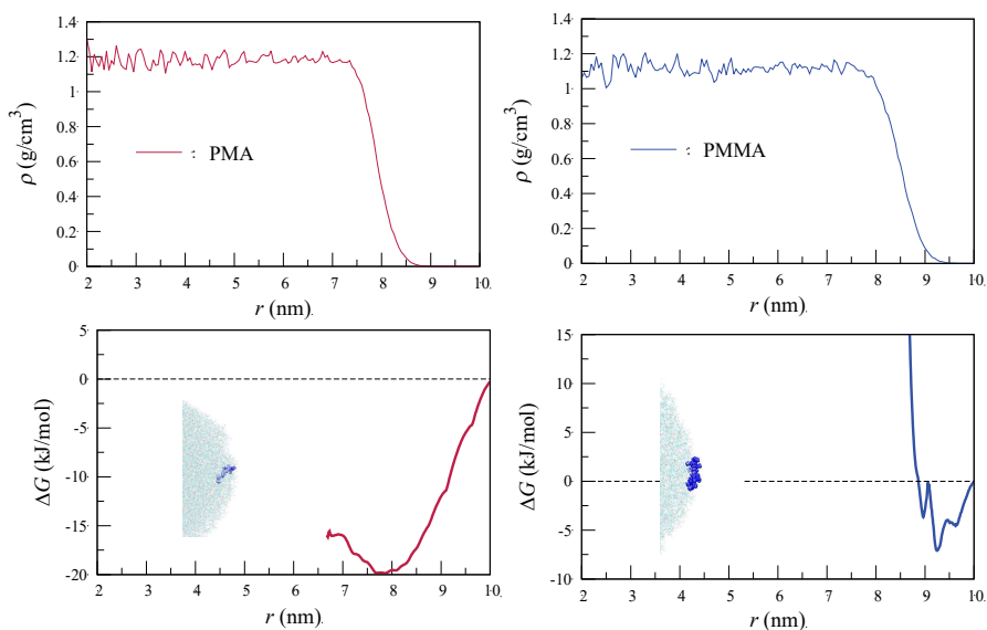
図 5. PMA (左) と PMMA (右) 微粒子の動径密度プロフィール (上段) と 10 量体の貫入自由エネルギープロフィール (下段)。
