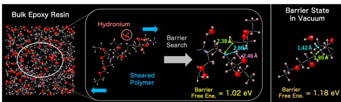
図 3. ずり応力を印加された硬化エポキシ樹脂に水分が侵入した状況の DFT-MD シミュレーション。水分に含まれる H_3O^+ が、プロトン化したアミン基に近づく際には、 1 \text{ eV} 程度の低いバリア自由エネルギーで、N-C ボンドが切断した。
