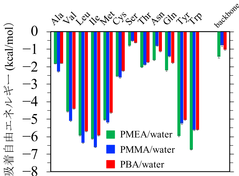
図 1. PMAA, PMMA, PBA の 3 つのポリマーと水の界面に対するアミノ酸アナログの吸着自由エネルギー。
