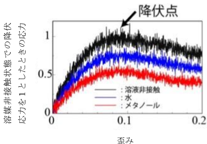
図 5. 水（青）またはメタノール（赤）と接触した系の応力歪み曲線と、接触していない系（黒）の応力歪み曲線。溶媒が接触していない場合の降伏応力が 1 となるように規格化している。
