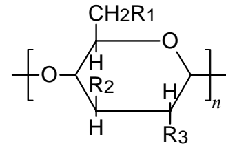
図 3. セルロースの構造。 R 1 , R 2 , R 3 が置換基であり、置換前には OH。
