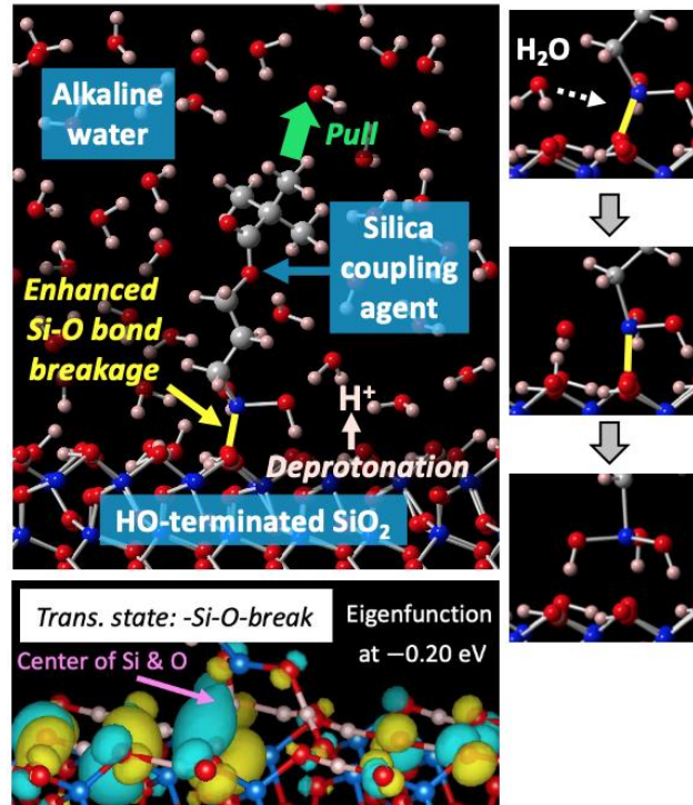
図 4. シリカカップリング剤を経て接着している樹脂/ \text{SiO}_2 界面に水分が侵入した状況のシミュレーション。中性あるいはアルカリ性の水分の場合、 \text{SiO}_2 表面は部分的に脱プロトン化して表面電子が生じ、さらに水分子の解離も相まって、カップリング剤と \text{SiO}_2 基板をつなぐ \text{Si-O} ボンドの破壊に関わるバリアエネルギーは大きく下がる。
