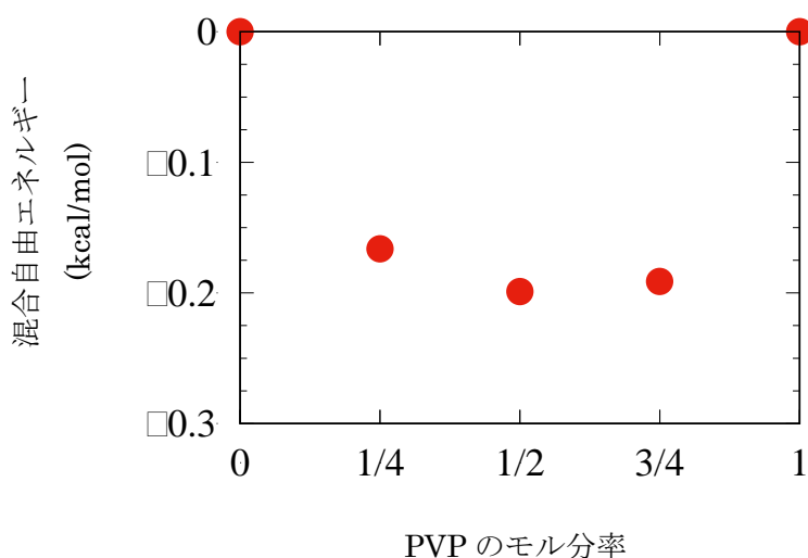
図 2. PVA と PVP の混合自由エネルギー。自由エネルギーは、モノマー1つ当たりの値。
