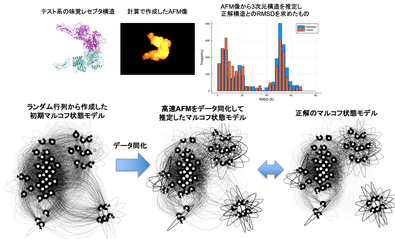
図2-1-2: テストデータを用いた高速AFMデータ同化の検証結果。
