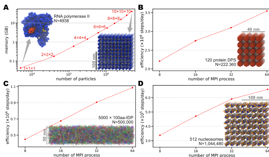
図1-1-5: GENESIS/ATDYNに導入されたAICG2+を用いたベンチマークテストの結果。
