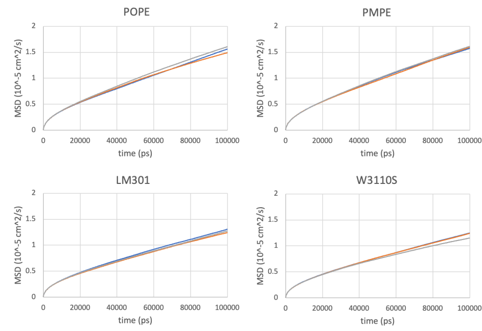
図3-5-3: Mean square displacement (MSD) の時間変化。3本のトラジェクトリによる結果を色分けした。
