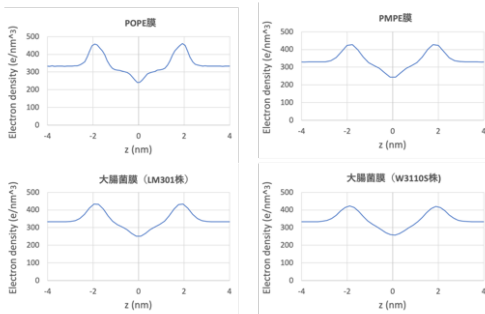
図3-5-2: 膜の電子密度プロファイル。横軸zは膜に垂直な方向を示す。膜の中心をz=0 とする。
