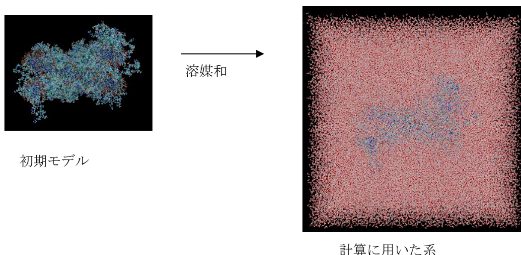
図3-3-6: フィッティングに用いられた水分子を含んだクロマチン結合因子GATA3とヌクレオソームが結合した複合体構造モデル。系の原子数は、複合体が約3万原子、水分子が約12万分子で、合計約39万原子である。系のサイズは 164\text{\AA} \times 164\text{\AA} \times 164\text{\AA} 。塩濃度は150mMとした。
