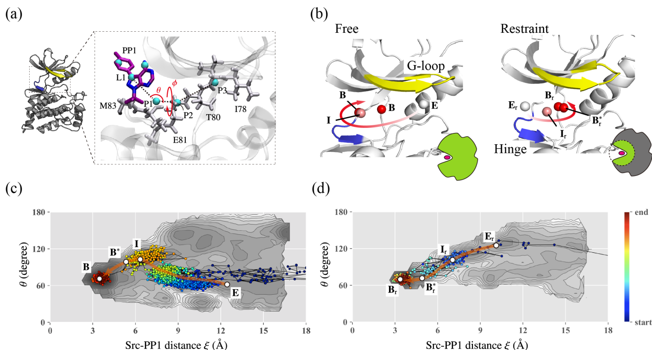
図 3-1-1: c-Src Kinase と阻害剤 PP1 の結合・解離シミュレーション。(a) タンパク質 c-Src Kinase と PP1 結合部位のクローズアップ。(b) 希薄溶液中およびタンパク質に拘束条件をつけないレプリカ交換法で観測された結合経路と、混雑溶液中およびタンパク質に拘束条件をつけたレプリカ交換法で予測した結合経路の違い。(c) 希薄溶液中（およびタンパク質に拘束条件をつけないレプリカ交換法）での自由エネルギー面と MD 計算での軌跡。(d) 混雑環境中（およびタンパク質に拘束条件をつけたレプリカ交換法）で得られた自由エネルギー面と MD の軌跡。
