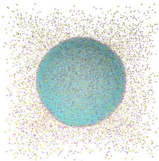
図1-2-8: 640万粒子のベシクル系。
