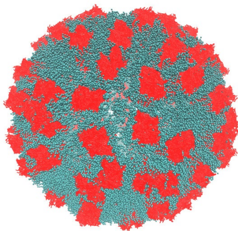
図3-4-6: POPC（空色）ベシクル中にS 2 量体（赤色）構造を140個埋め込んだ状態の構造。 重なりのある脂質分子を削除したため局所的に脂質分子が疎なところが生じている。
