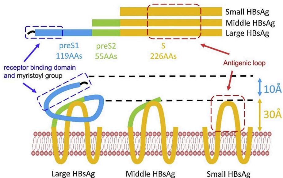
図3-4-1: B型肝炎ウイルスのエンベロープタンパク質3種類 Small (S), Middle (M), Large (L) の比較。上はアミノ酸配列の比較。下は膜貫通領域が共通で、細胞外領域に違いがあることを示している。Cao et al. , Virus Research , 2019 より改変。
