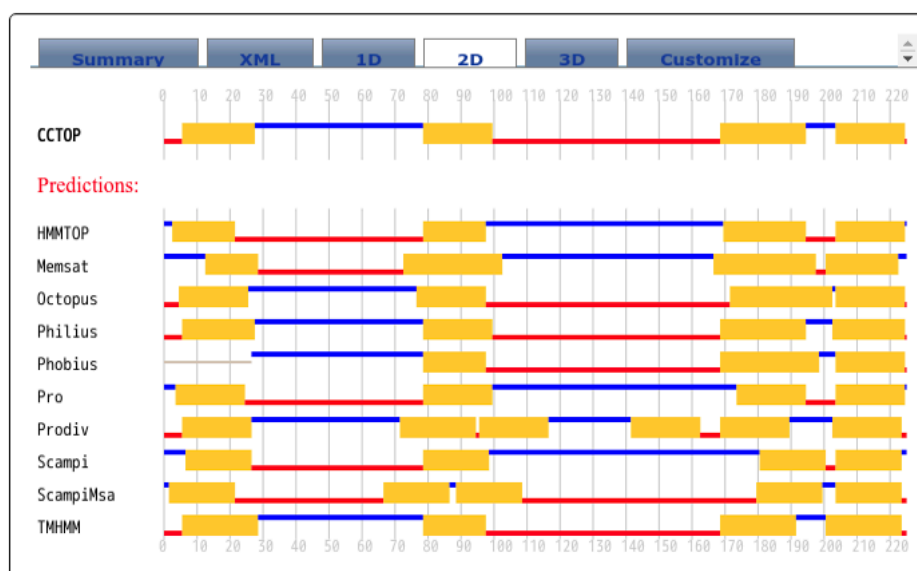
図3-4-2: 膜タンパク質の膜貫通領域予測構造サーバーConstrained Consensus Topology (CCTOP) より、HBV S タンパク質の構造予測の結果。黄色の領域が膜貫通領域を表し、青が膜外内側、赤が膜外外側を示している。一番上のCCTOPが最終的な予測配列である。
