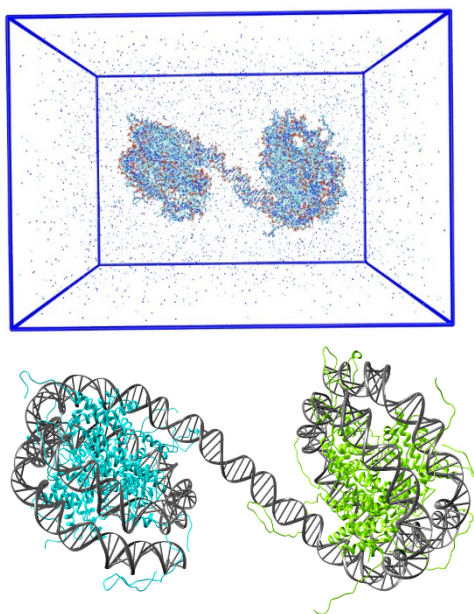
図3-3-4: ヌクレオソームダイマーの系（約100万原子）。全体の系（上図）とヌクレオソームダイマーのリボンモデル表示（下図）。
