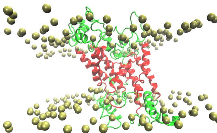
図3-4-5: 真空中で得た2量体構造を脂質二重層膜に入れて30 nsのMDシミュレーションを行った後の構造。黄色の分子は脂質頭部のリン原子である。その他の脂質の原子、水、イオンは省略した。
