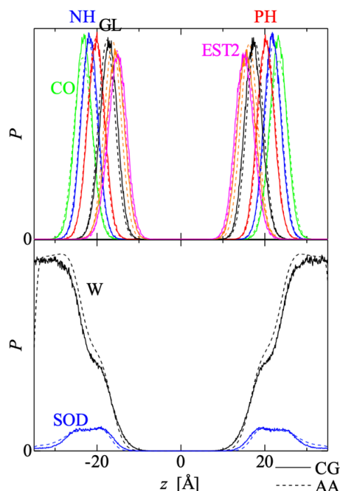
図1-2-4: 膜垂直軸に沿っての各粗視化セグメントの分布。脂質のセグメント名は図1-2-1に対応している。SODは水和ナトリウムイオン( \text{Na}^+(\text{H}_2\text{O})_3 )、Wは水( (\text{H}_2\text{O})_3 )である。
