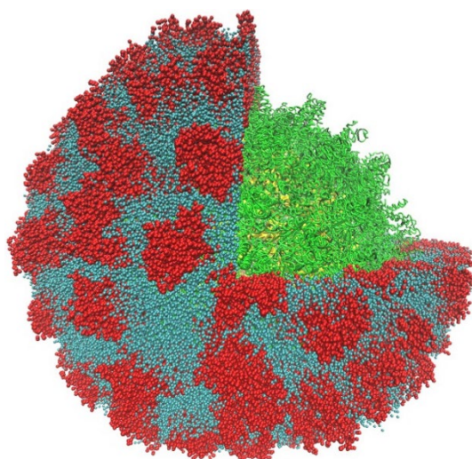
図 3-4-8: S2量体(赤色)を含んだエンベロップ構造に対して、内部にRNA(黄色)含有カプシド(緑色)を配置したスナップショット。内部構造を表示するため、エンベロップの1/4を非表示にした。
