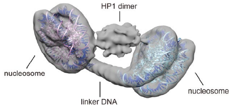
図3-3-1: ヌクレオソームとHP1の電子顕微鏡像。
