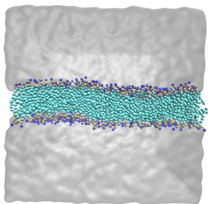
図1-2-7: DMPC脂質膜系のスナップショット。灰色は水分子領域、脂質分子は球で表示。
