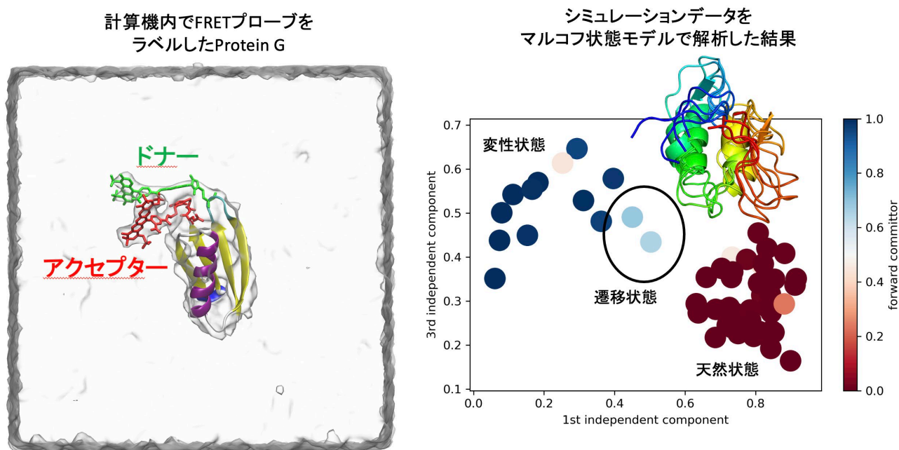
図2-1-3: Protein Gの構造サンプリング (MDシミュレーション) によって得られたマルコフ状態モデリング。
