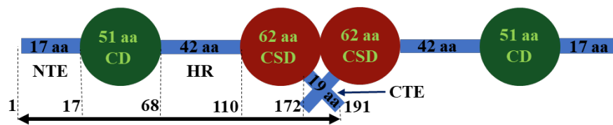
図3-3-2: HP1のトポロジー。
