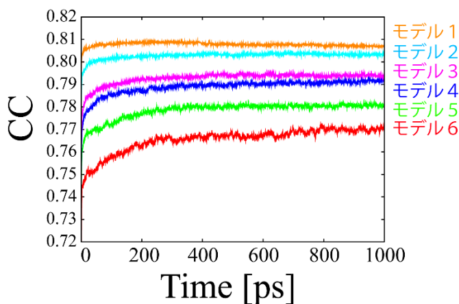
図3-3-7: MDシミュレーションによるフィッティング。横軸はシミュレーション時間、縦軸は電子密度に対する相関係数(CC)。CC=1.0のとき、複合体の立体構造から計算される理論的電子顕微鏡像と完全に一致する。MDシミュレーションはCCがほぼ一定値となる1 nsまで実施。モデル1から6は、フィッティング力 100k, 50k, 20k, 15k, 10k, 5kに対応。
