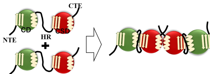
図3-3-3: 推定されたHP1ダイマー構造。
