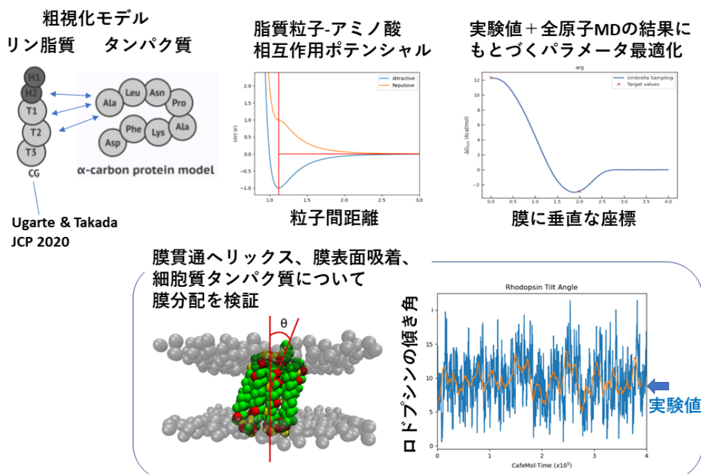
図2-2-1: 脂質分子の新しい粗視化分子モデルの開発。
