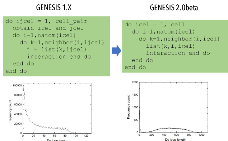
図1-1-1: GENESISにおける非共有結合相互作用計算のアルゴリズム。
