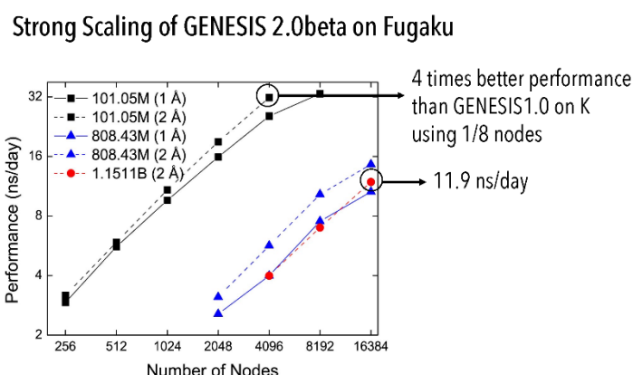
図1-1-3: GENESIS2.0betaを用いて実施した「富岳」上での巨大生体分子系のMDシミュレーションのベンチマーク結果。粒子数が増えた場合も効率的な計算ができていることを示す。
