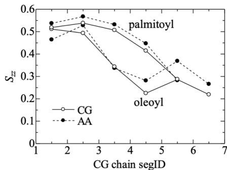
図1-2-3: 疎水鎖のオーダーパラメータ。
