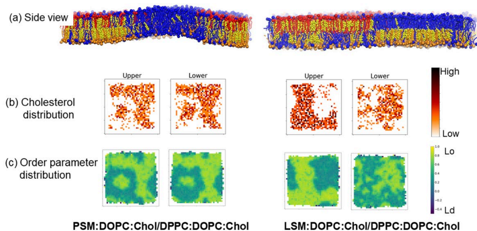
図1-2-6: 上下層とも相分離する膜の層間相互作用。PSM系とLSM系の比較。(a)側方スナップショット、(b)上下層のChol分布、(c)オーダーパラメータ。
