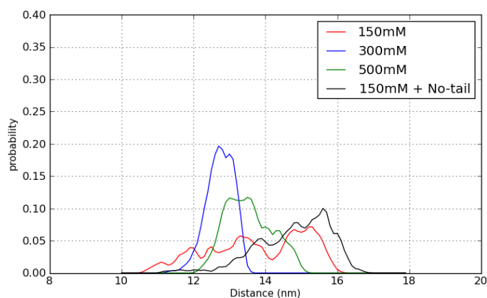
図3-3-5: 2つのヌクレオソームの重心間距離分布。 テール有の系では、塩濃度 150, 300, 500 mM で計算を実施。 テール無の系では、塩濃度 150mM で実施。
