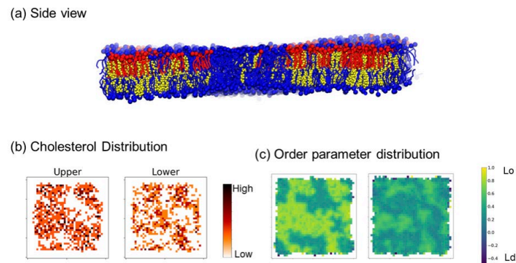
図1-2-5: PSM(赤)/DOPC(青)/Chol(黄)のMDからの(a)スナップショット、(b)上下脂質層におけるCholの分布、(c)上下層における脂質のオーダーパラメータ。
