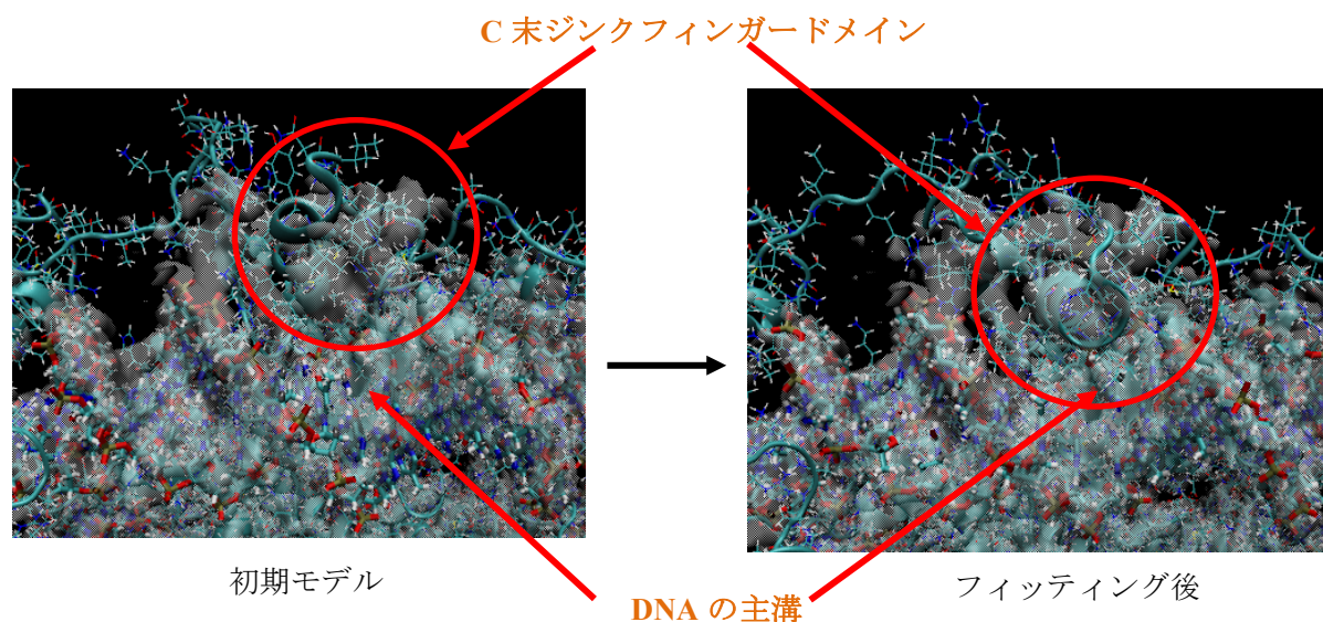
図3-3-8: MDシミュレーションにより構築された複合体モデル。初期モデルでは、GATA3のC末ジンクフィンガードメインが電子顕微鏡像から大きく外れている。フィッティング後には、C末ジンクフィンガードメインが電子顕微鏡像にフィットし、DNAの主溝と相互作用するようになった。
