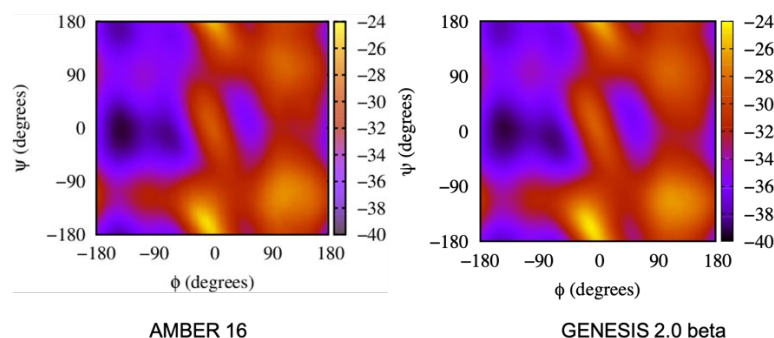
図 1-1-6: GENESIS2.0beta および AMBER16 を用いて Alanine-dipeptide に対して実施した ABMD 計算の結果。φ、ψ の 2 次元自由エネルギー面がよく一致していることを示す。
