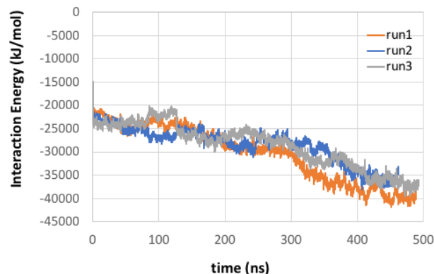
図3-5-5: 多剤排出トランスポーターAcrAB-To1C複合体と大腸菌モデル膜との相互作用。 初期運動量を変えた3つのシミュレーションの結果を表示している。
