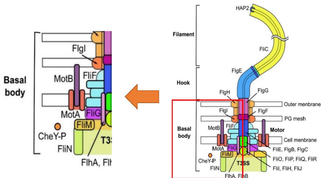
図3-1-2: 細菌べん毛の全体構造の模式図（右）と固定子付近の拡大図（左）。
