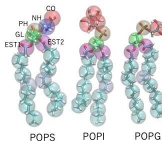
図1-2-1: POPS, POPI, POPGの粗視化モデル(球)。対応する全原子モデルはstickで表示している。各粒子の定義はCO: -\text{CO}_2^- , NH: -\text{CH}(\text{NH}_3^+)\text{CH}_2- , PH: -\text{PO}_4^- , GL: -\text{CH}_2\text{CH}=\text{CH}_2- , EST1/EST2: -\text{CCO}_2^- 。
