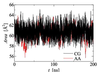
図1-2-2: POPS膜の膜面積変化。
