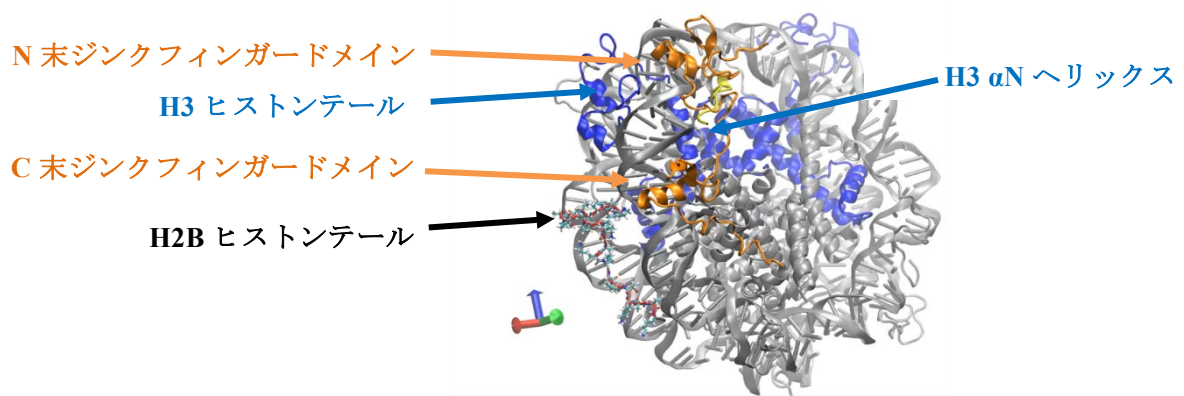
図3-3-9: GATA3 (リボンモデル、橙色) のN末ジンクフィンガードメインがH3ヒストンテールと、C末ジンクフィンガードメインがH2Bヒストンテールと相互作用する様子。H3ヒストンテールはリボンモデル、青色で表示、H2Bヒストンテールは原子モデル、主鎖を赤色で表示。
