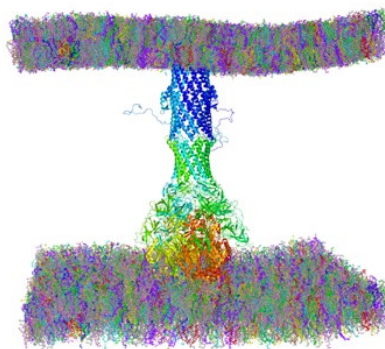
図3-5-4: 大腸菌モデル膜に埋め込んだ多剤排出トランスポーターAcrAB-TolC複合体。大腸菌モデル膜は脂質分子の種類によって色分けして表示している。
