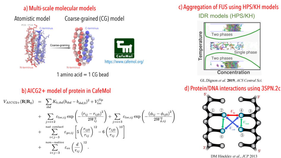
図1-1-4：粗視化分子モデルの説明。a) 全原子モデルと粗視化モデルでの粒子の取り扱いの違い。b) CafeMolのタンパク質モデルAICG2+で用いられているエネルギー関数。c) 天然変性タンパク質を扱う粗視化分子モデルHPS/KH。d) 核酸に適用される粗視化分子モデル3SPN. 2c。
