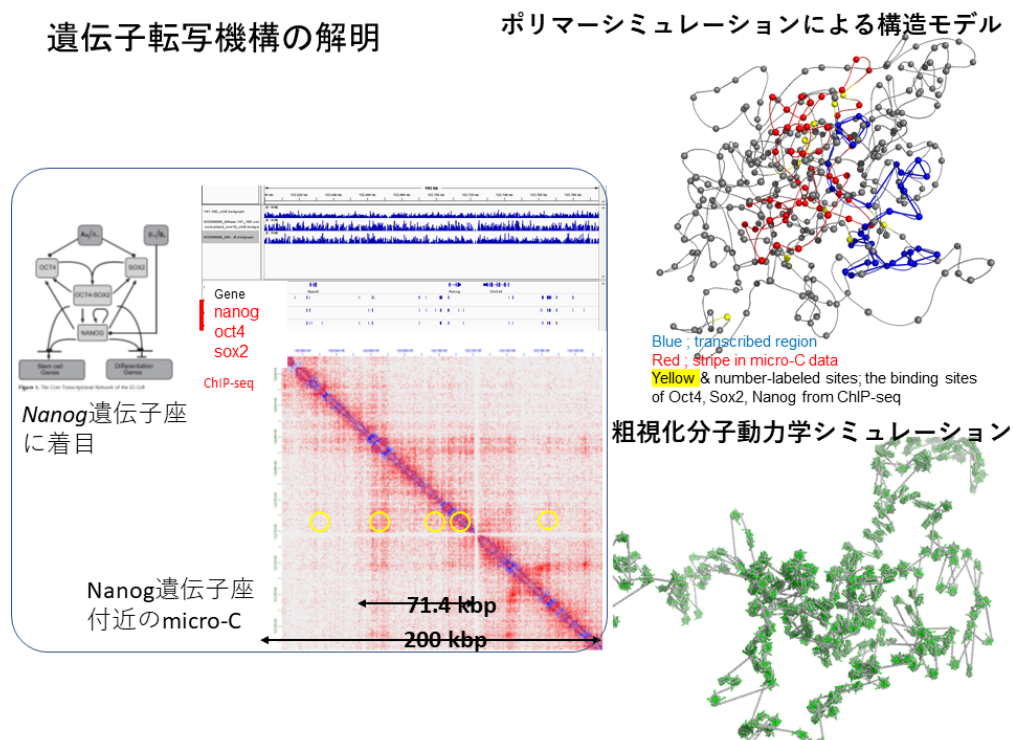
図3-2-1: 遺伝子転写機構の解明にむけた生体分子系モデリングとシミュレーション。
