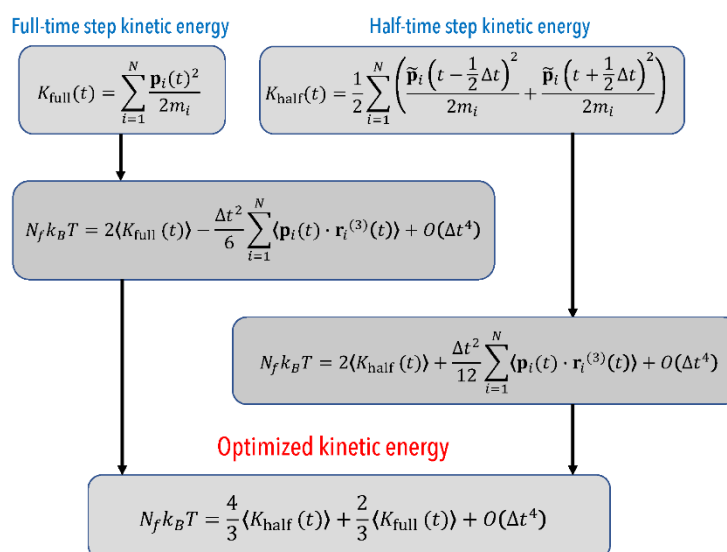
図1-1-2: MDシミュレーションにおける運動エネルギーの定義。
