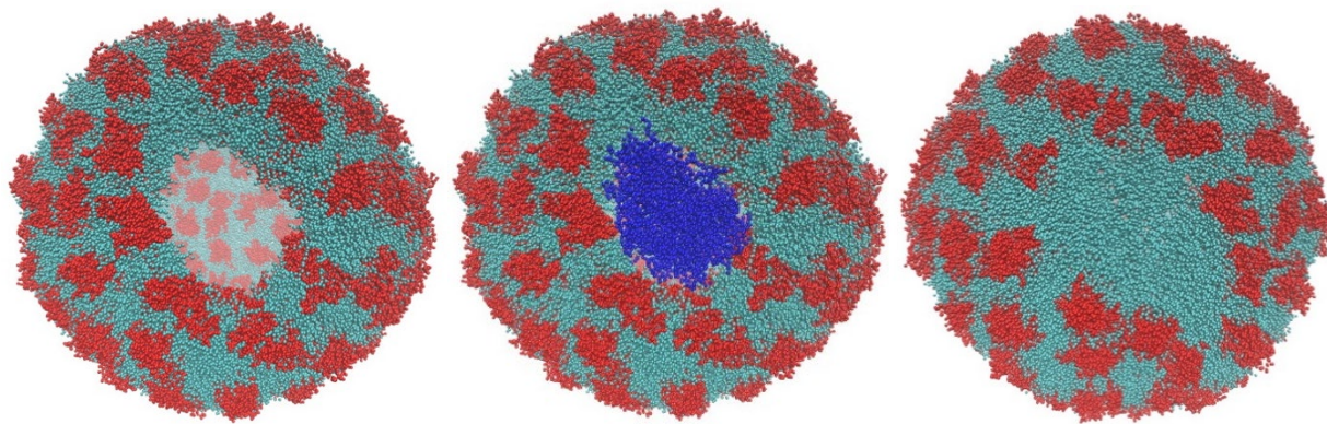
図3-4-7: (左)埋め込み後、30 nsの平衡化MDシミュレーションを行った後の構造。脂質膜に細孔が形成されている。(中) 細孔部分に、脂質パッチ(青色)を追加した状態。(右) 脂質パッチの配置後、再度、平衡化MD計算を30 ns行ったあとのスナップショット。細孔のないエンベロップ構造が作成された。
