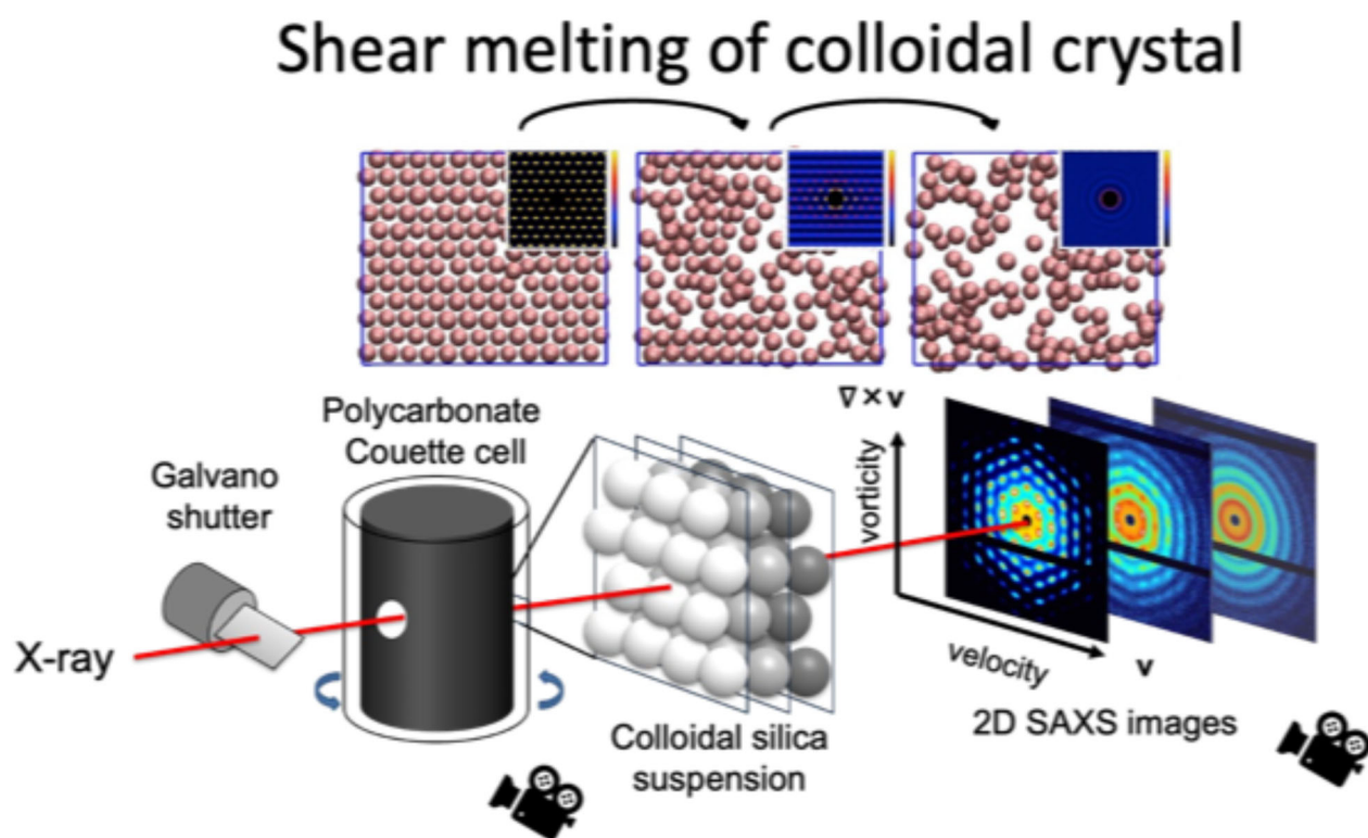
図1 コロイド結晶のせん断融解と時間分解 rheo-SAXS/USAXS 測定システムの概要。
